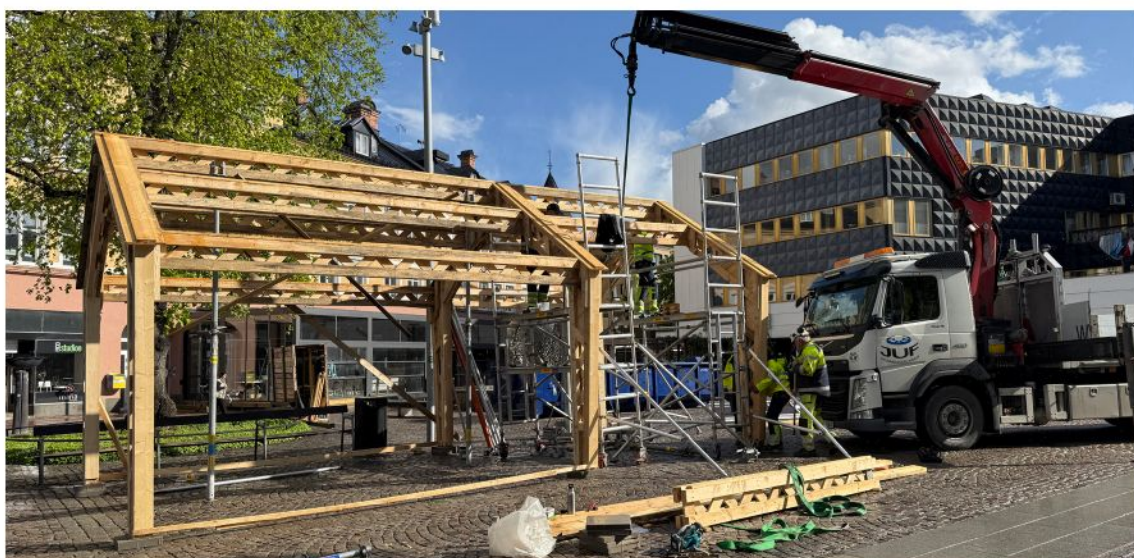
Montering och resning av paviljongen på Sveatorget. Foto: Gaia ark
